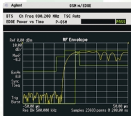
EDGE power versus time
