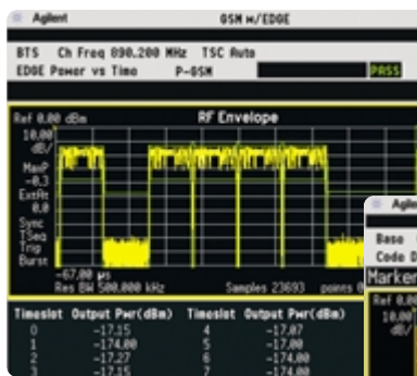
EDGE power versus time
